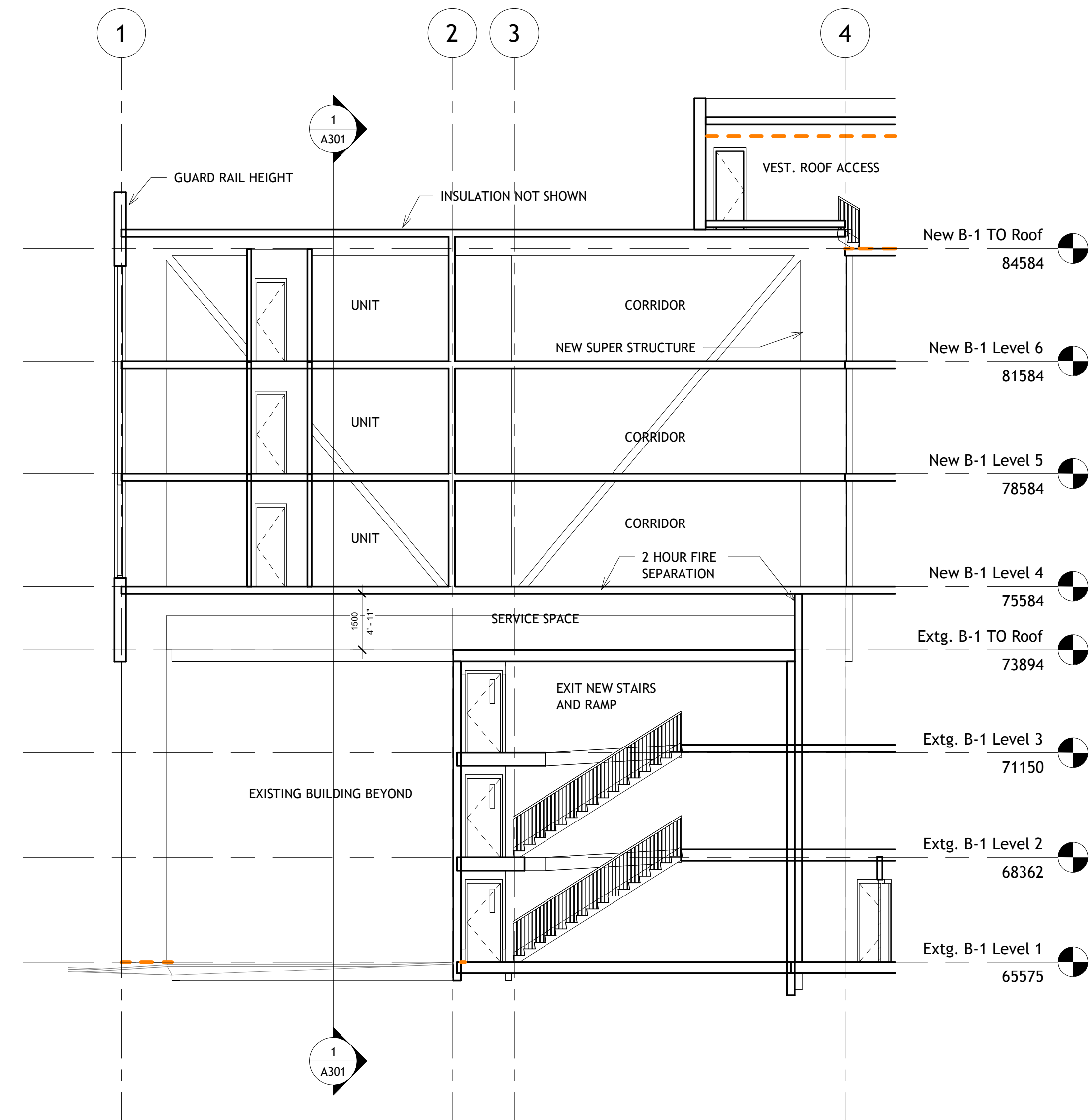
2 Bldg 1 section 2 1 : 100
