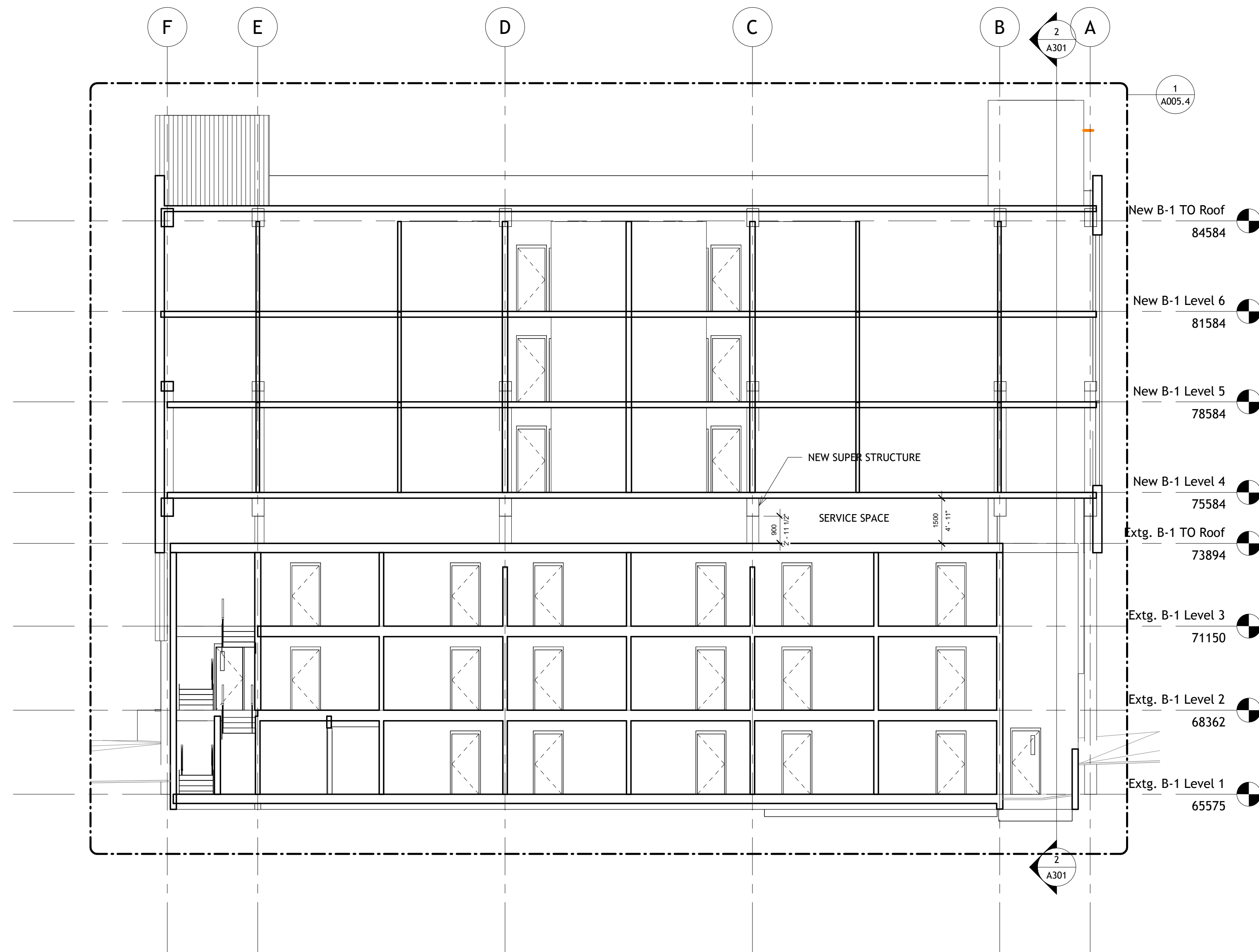
1 Bldg 1 Section 1 1 : 100
